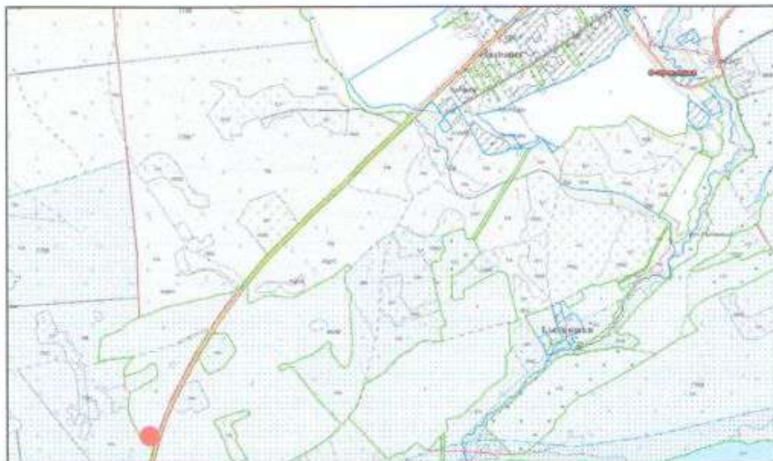
Схематическая карта (план) геологического памятника природы местного значения «Видинский валун»
